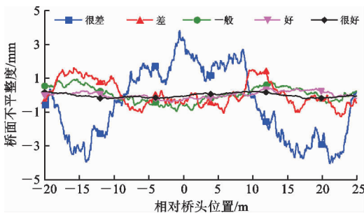
图 5 桥面不平整度曲线
