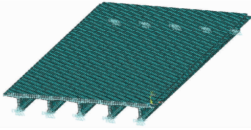
图 2 T20 桥梁有限元模型
