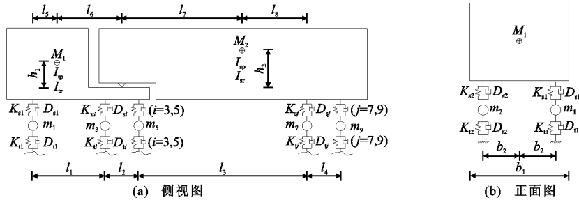
图 3 车辆模型示意
